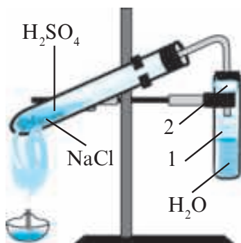
Рис. 75. Дар лаборатория ҳосил кардани кислотаи хлорид;
