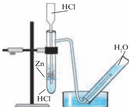
Рас. 42. Ҷамъ кардани гидроген бо усули фишурда баро ҷардани об
