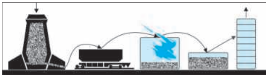
Рас. 56. Ҳосил кардани оҳаки шукуфта: 1) шикта (оҳаксанг ва сӯзишворӣ); 2) шукуфонидани оҳаки пухта; 3) рег; 4) об; 5) бинои хиштин.
