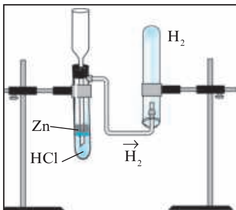
Рас. 44. Ҷамъ кардани гидроген бо усули фишурда баровардани ҳаво
