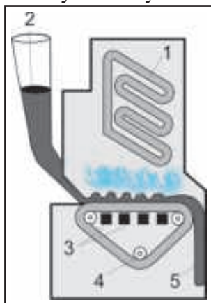
Рас. 39. Сӯхтани сӯзишвори сат: 1-қубурҳои обдор, 2-сузишворӣ, 3-панҷара, 4-сӯрохи ба рои ҳаво, 5-двэгол.
