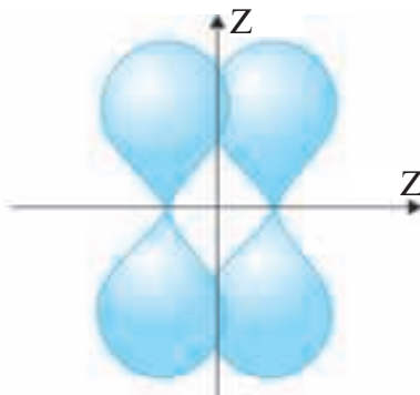
Расми 62. Ҳосил шудани \pi банд
