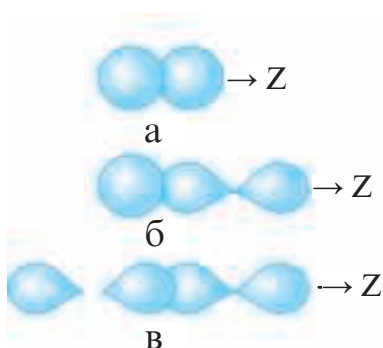
Расми 61. Ҳосил шудани \sigma банд дар натиҷаи рӯйпӯш шудани: а) s-s, б) s-p, в) p-p абрҳои электронӣ
