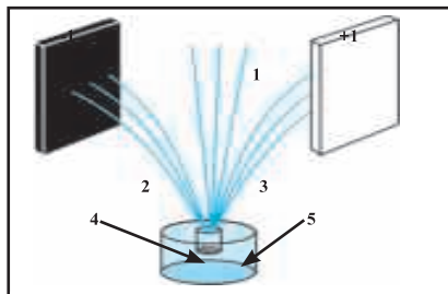
Рас. 57. Таҷзияи нурҳои афканишоти радиоактивӣ дар майдони барқӣ
