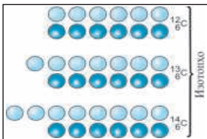
Рас. 58. Таркиби ядрои атоми изотопи карбон (даврачаҳои сирёхпротонҳо, даврачаҳои кабуди нейтронҳо)
