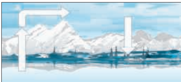
Рас. 53. Се ҳолати агрегатии об дар табиат: ях (барф) дар қўҳҳо, оби моеъ дар қўлҳо, абрҳо дар атмосфера
